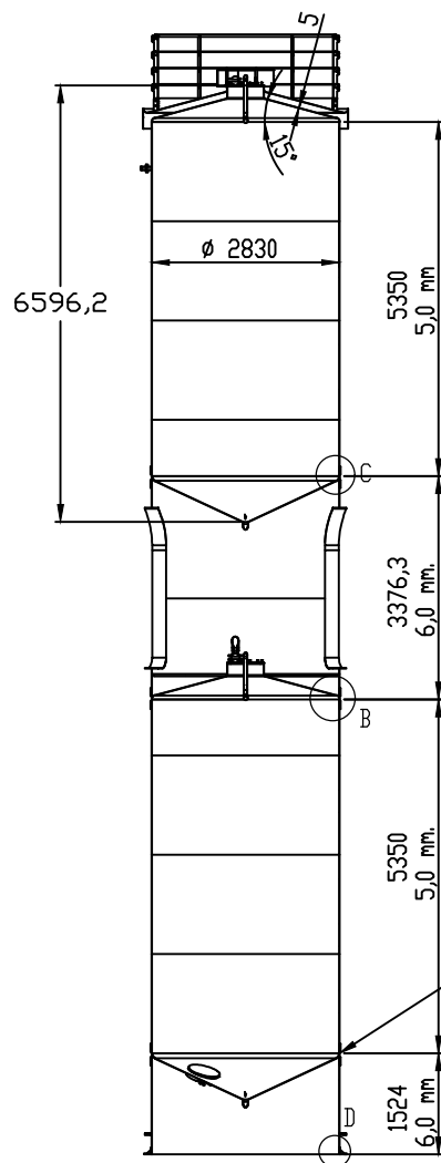
SECTION A-A
